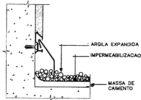
ARREIMATE DE BORDAS LATERAIS DE IMPERMEABILIZACAO
