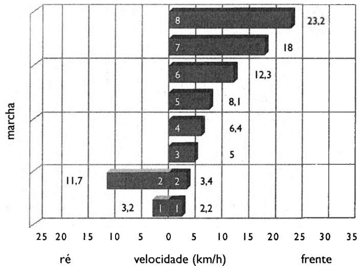
ESCALONAMENTO DE MARCHAS
