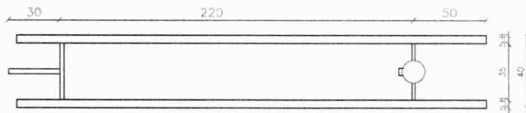
PLANTA BAIXA
