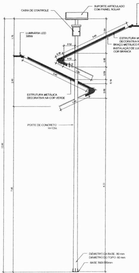
VISTA FRONTAL ESCALA 1:50
