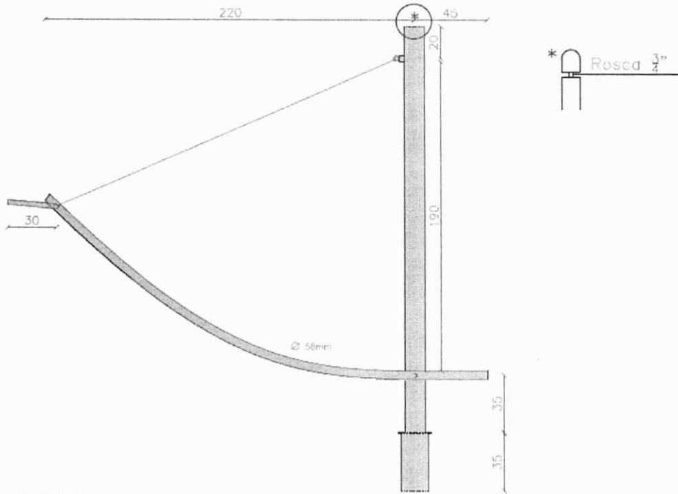
VISTA LATERAL
