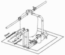
DETALHE DO ESQUEMA DE BOMBA ESCALA 1:50
