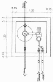
PLANTA BAIXA CASA DE MÁQUINAS ESCALA 1:50
