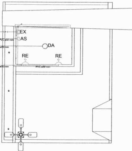
PLANTA BAIXA HIDRÁULICA ESCALA 1:50
