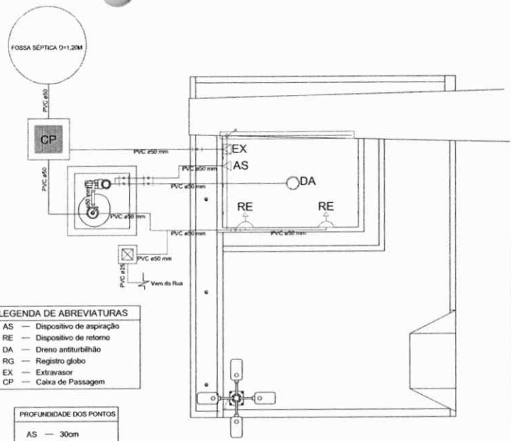
PLANTA BAIXA HIDRÁULICA ESCALA 1:20
