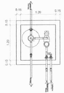
PLANTA BAIXA CASA DE MÁQUINAS ESCALA 1:20
