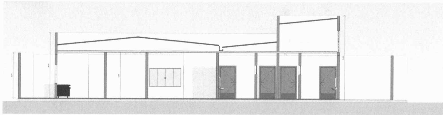
1 CORTE A 1 : 35
